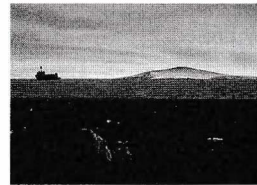
19. Ocean Planet
