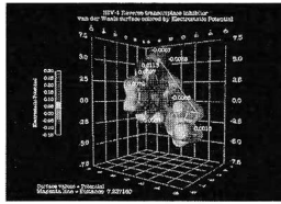
32. HIV
