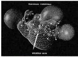
31. Molmine
