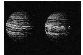
15. Jovian Planet
