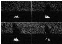
11. Bonfire
